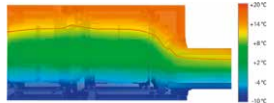
Isothermenverlauf ADS 90 SimplySmart
